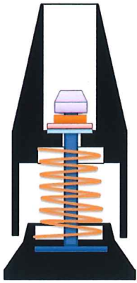
断面図
